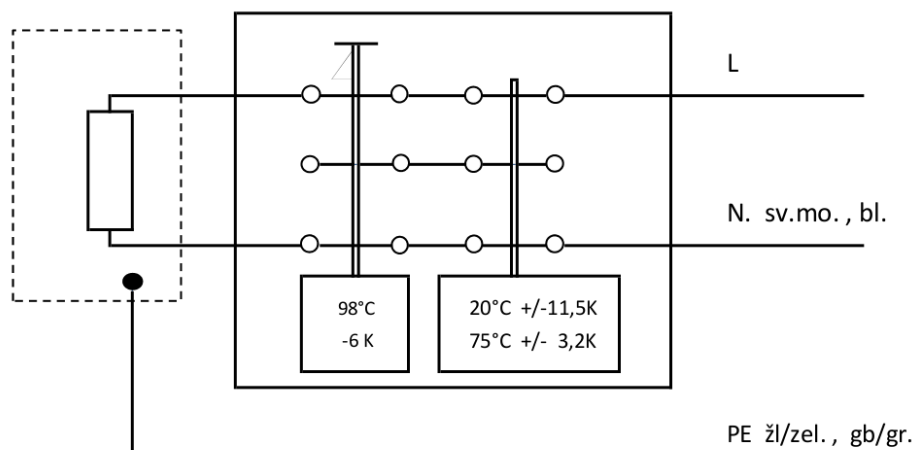
Schéma zapojení 1f
